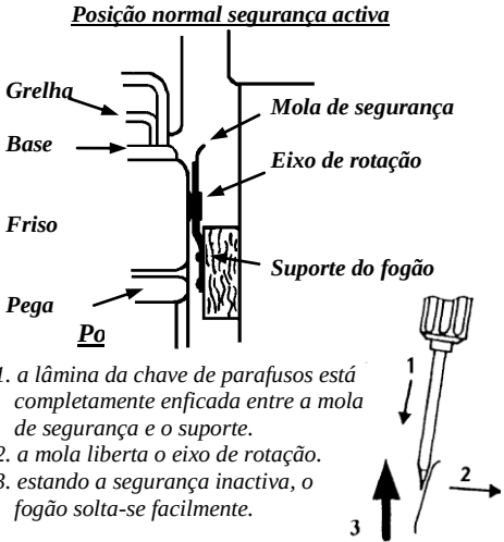
Esquemas: funcionamento da barra anti-oscilação
