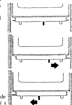
Schémas: fonctionnement de la barre anti-roulis.
